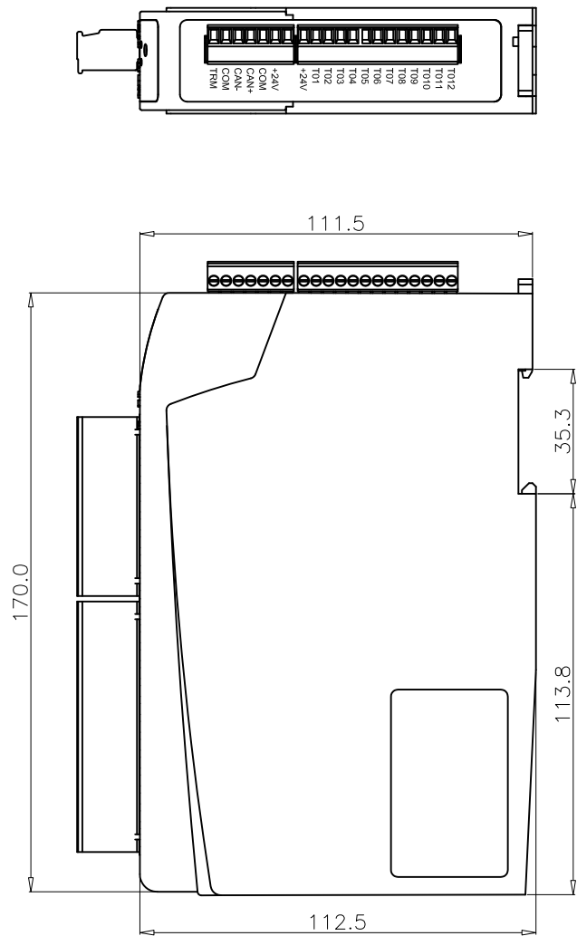
RMTP12 塑殼 安裝與外型尺寸圖
